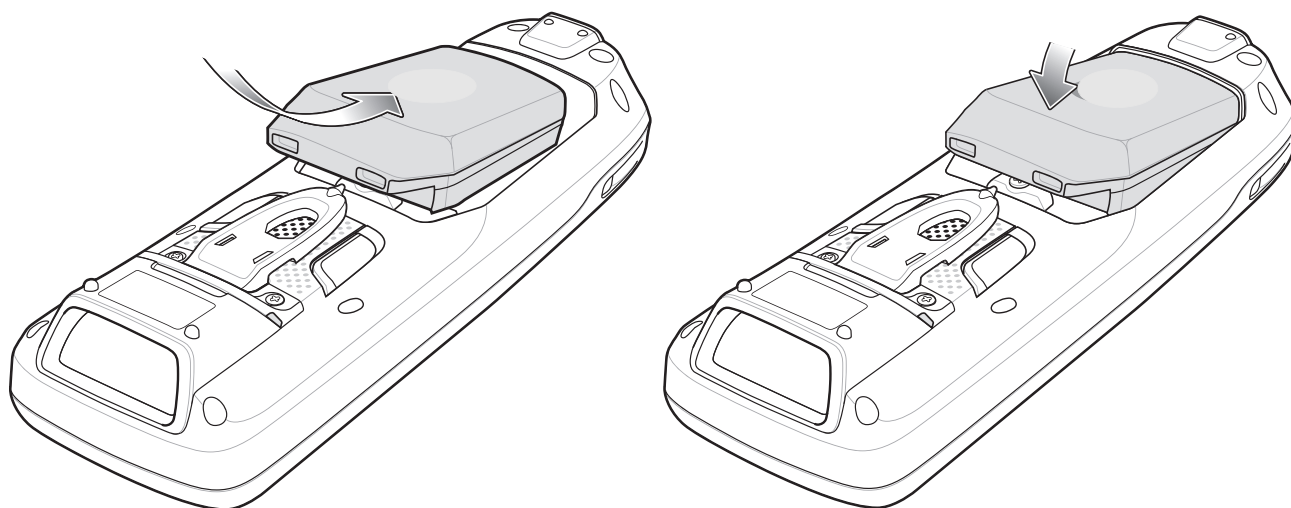
Рис. 1-4 Установка аккумулятора
