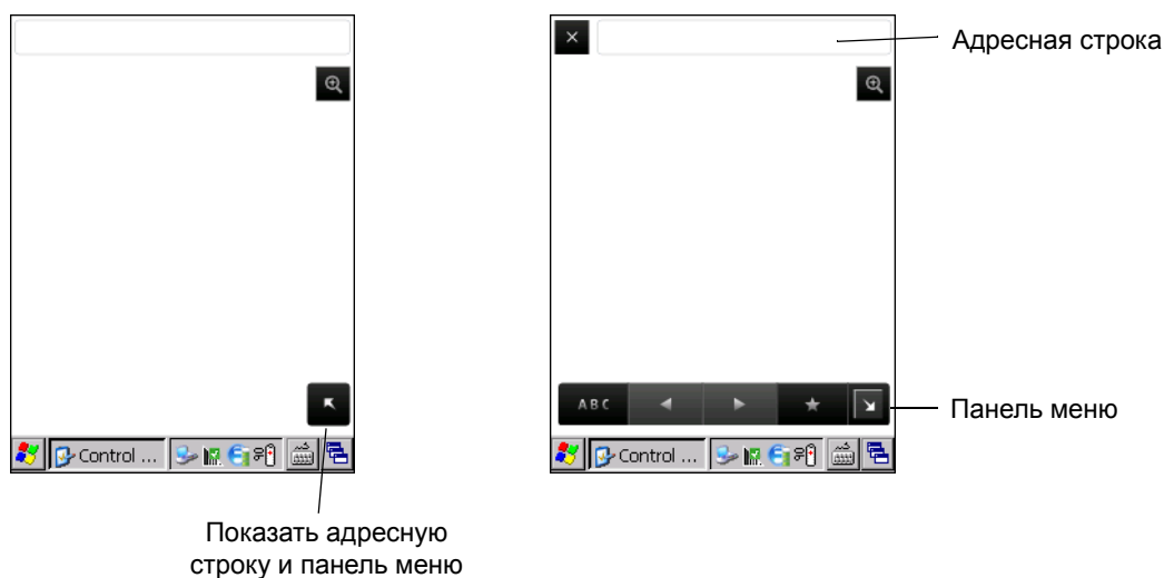
Рис. 2-15 Браузер
