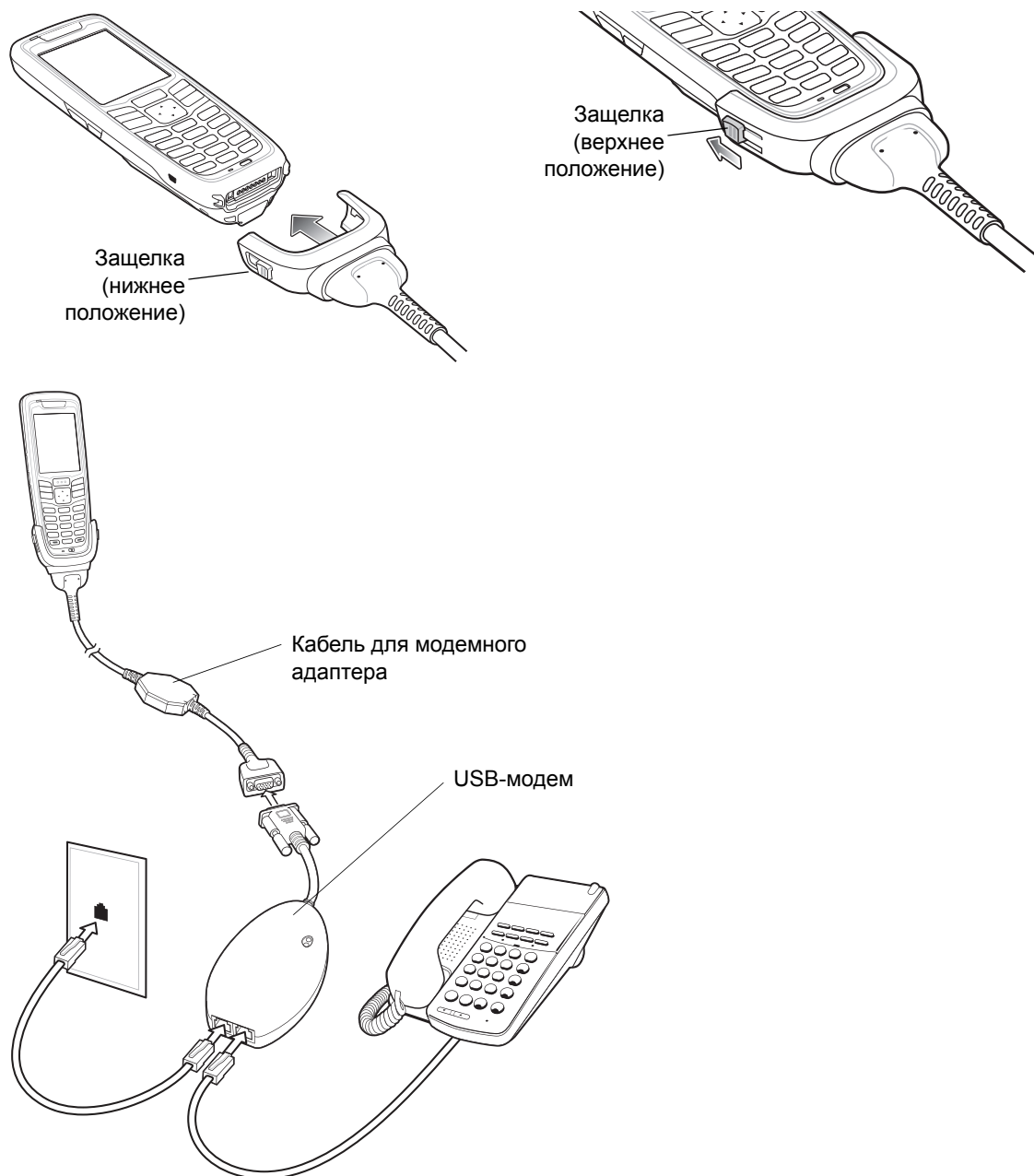
Рис. 6-7 Настройка USB-модема
